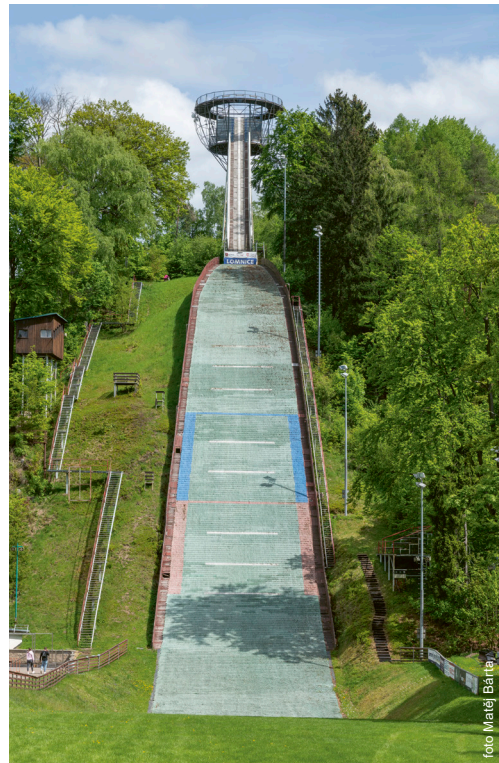
Skokanský můstek K70 s vyhlídkovým ochozem
